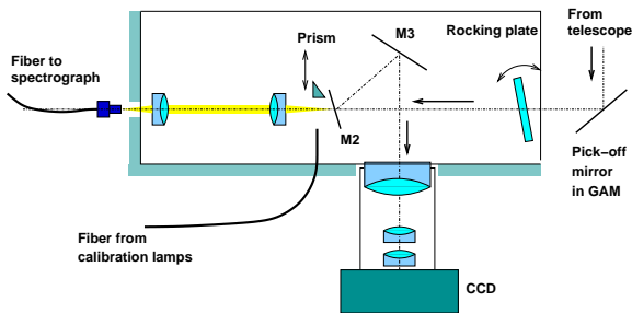
Fig. 3.— Fiber feed of CHIRON.
