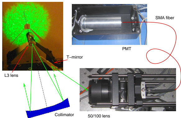
Fig. 4.— Exposure meter.
